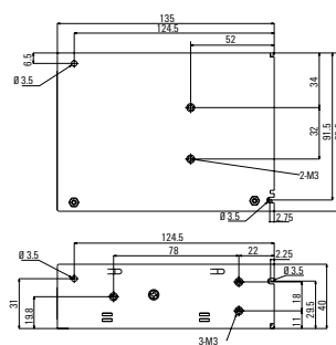
75W电源安装尺寸示意图
