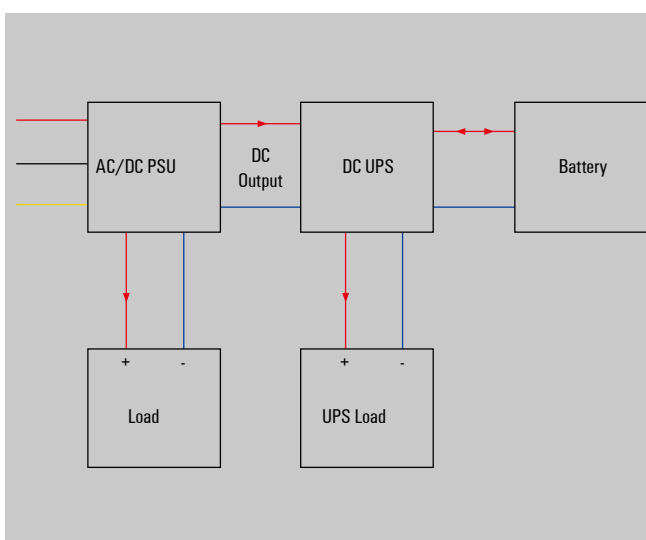
图(2) DC UPS系统
