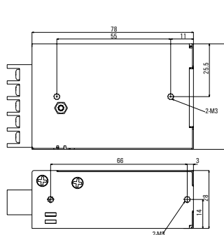
25W电源安装尺寸示意图
