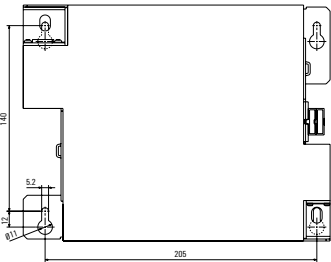
17Ah平面安装尺寸图
