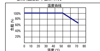
25W电源温度降额曲线
