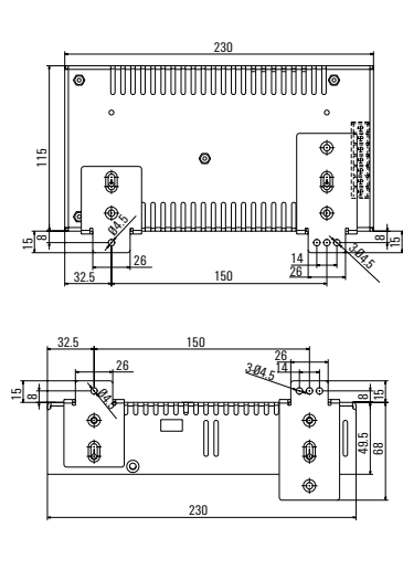
250W/350W电源安装尺寸示意图(带安装附件)
