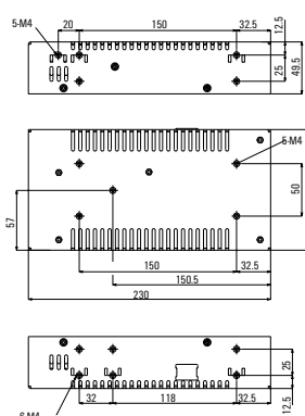
250W/350W电源安装尺寸示意图 (不带安装附件)
