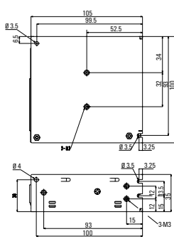
50W电源安装尺寸示意图
