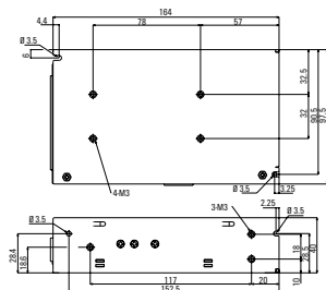
100W电源安装尺寸示意图
