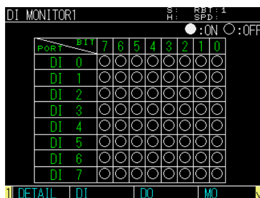
“DI 监控 1”画面
