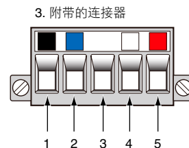
端子排列表
