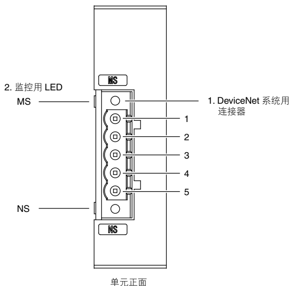
端子排列表
