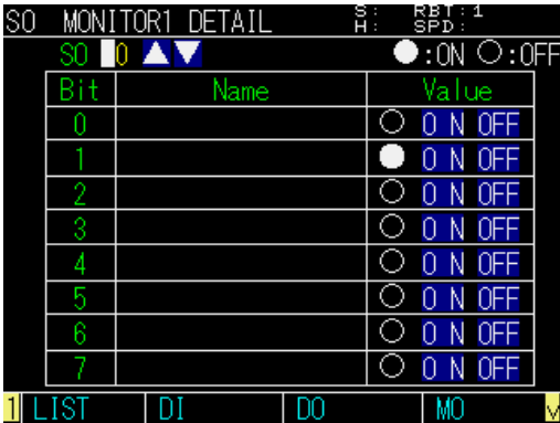
“SO 监控 1 详细”画面
