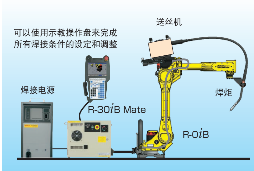
使用 R-0iB 的弧焊机器人系统
